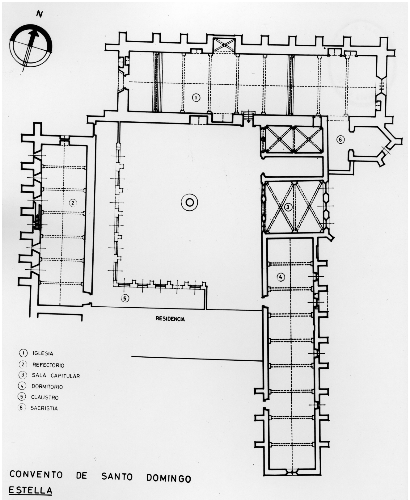
1. Planta del convento de Santo Domingo de Estella.
